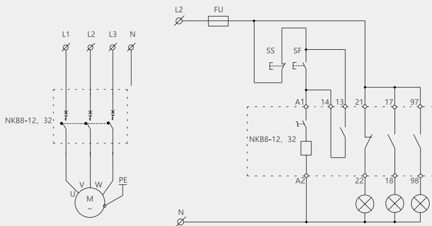
NKB8-12、32基本方案控制电路图2
