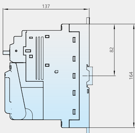
高级型导轨安装
