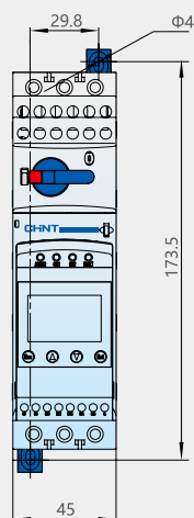
多功能型螺钉固定
