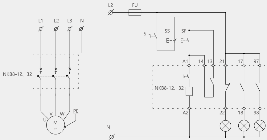
NKB8-12、32基本方案控制电路图1
