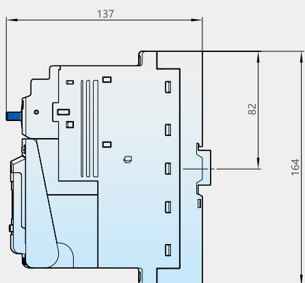
多功能型导轨安装
