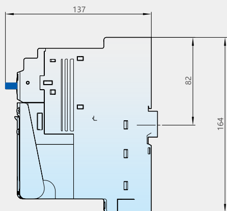
标准型导轨安装
