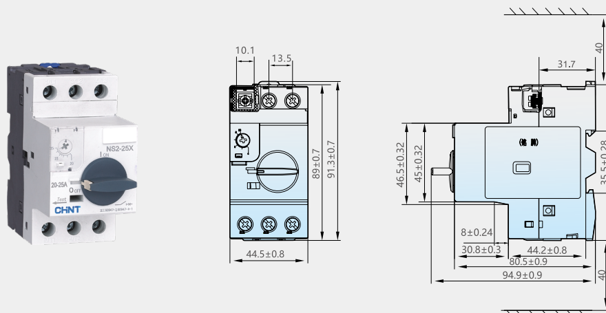
NS2-25X、NS2-32X起动器外形及安装尺寸
