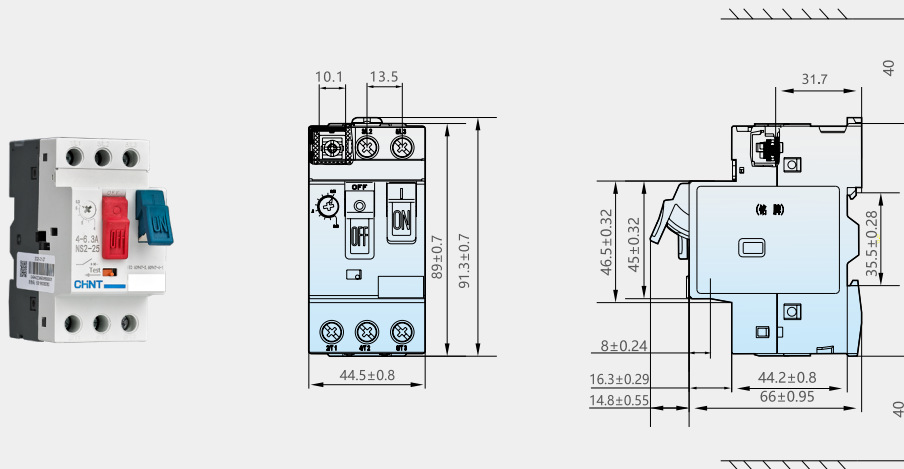
NS2-25、NS2-32起动器外形及安装尺寸
