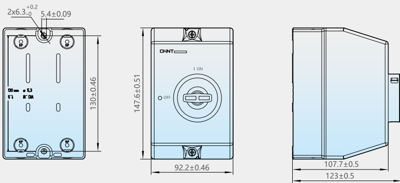
NS2-32H 起动机外形及安装尺寸
