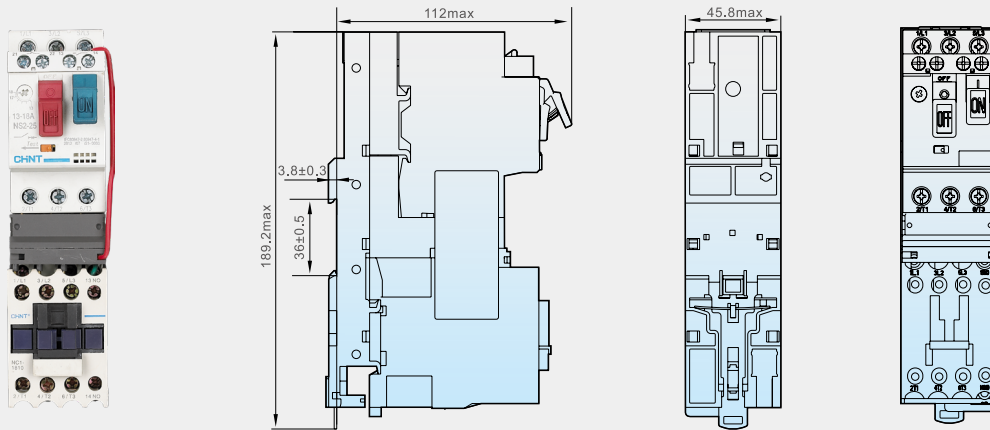
NQB1-18/BO标准型
