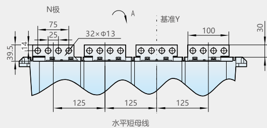
水平短母线
