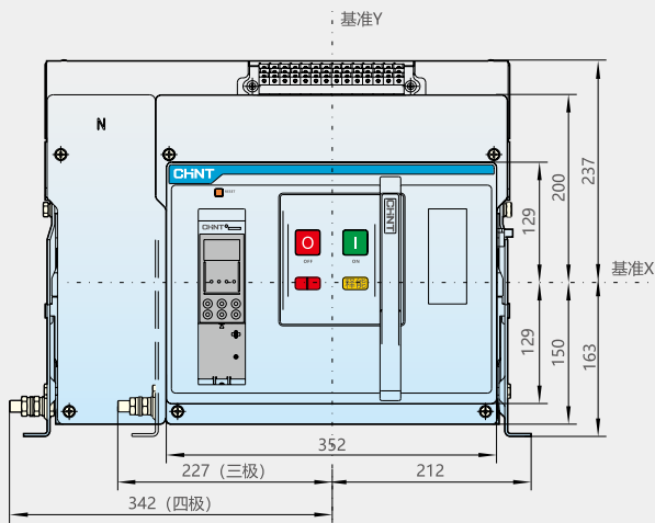
正面图
