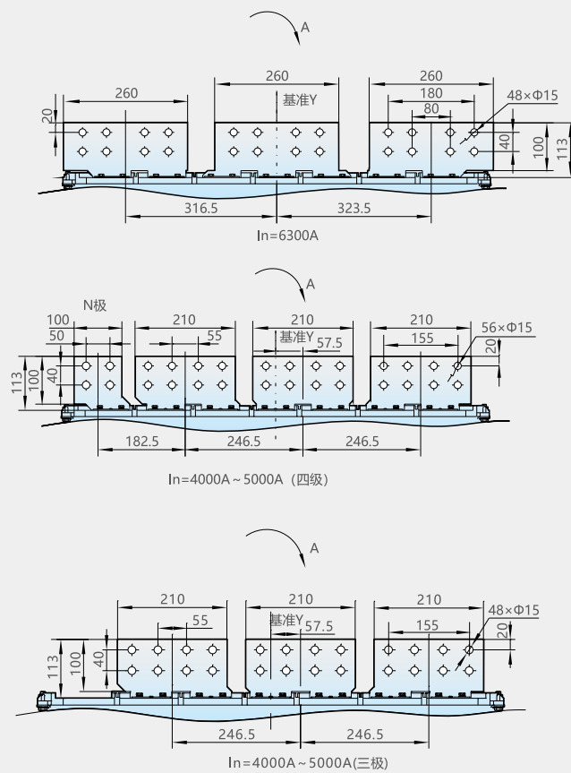
排尺寸及排间距
