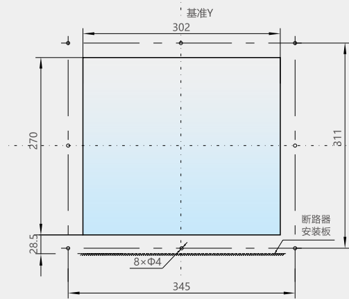
面板开孔
