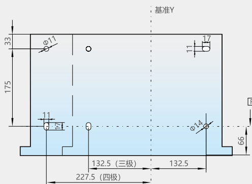
底座外形尺寸及安装孔距示意图
