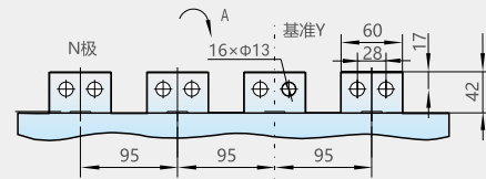
水平接线 (默认配置)
