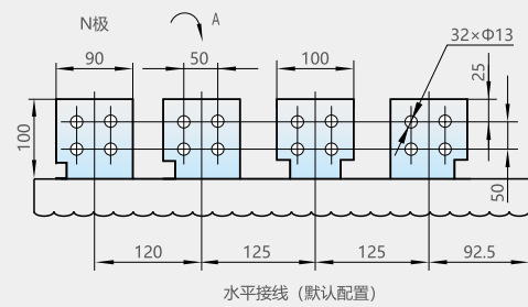
水平接线 (默认配置)
