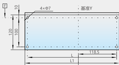
底座外形尺寸及安装孔距示意图
