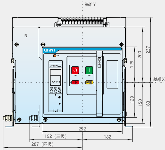
正面图
