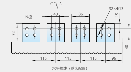
排尺寸及排间距
