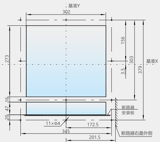
面板开孔
