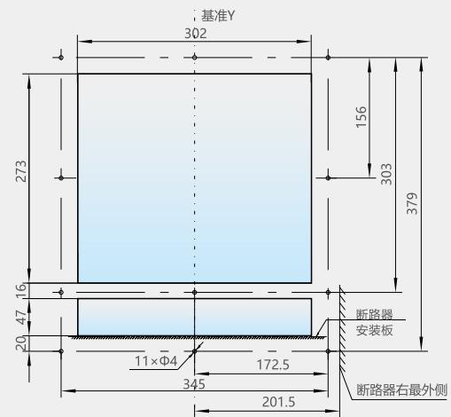
面板开孔
