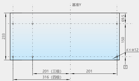
底面外形尺寸及安装孔距示意图
