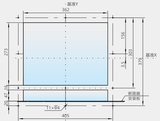
面板开孔
