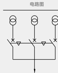
MI-4三联锁电路图
