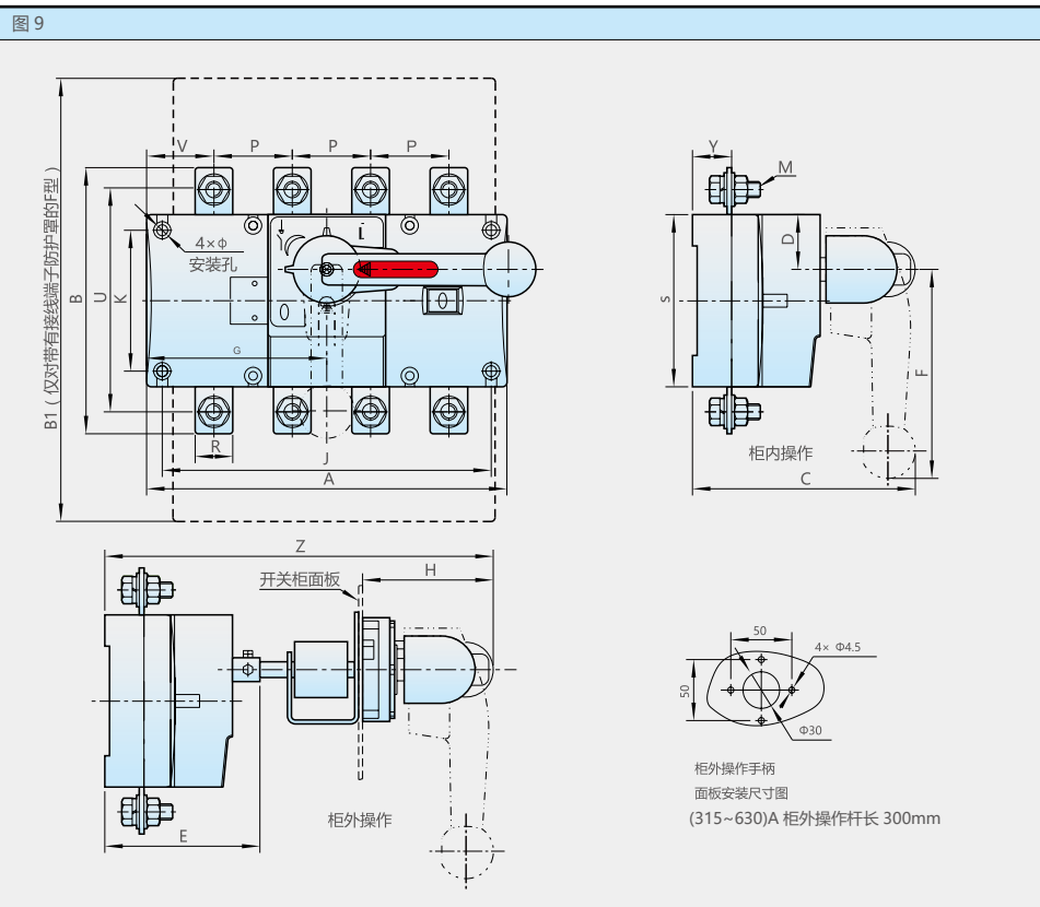
6.7 125A~630A 隔离开关外形及安装尺寸
