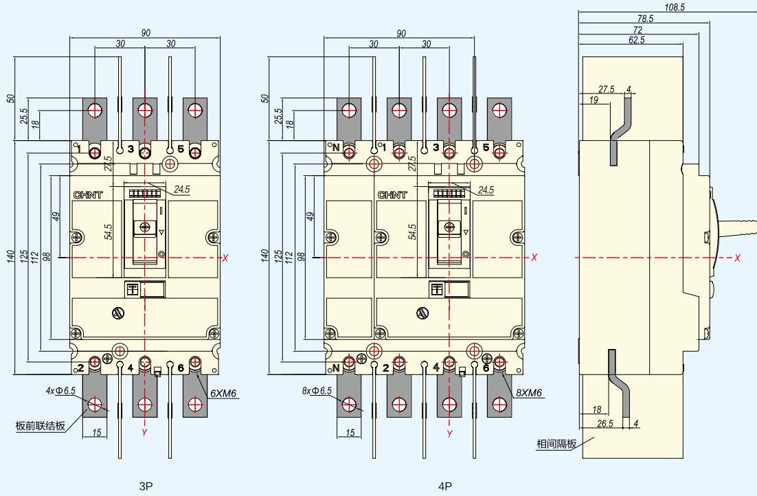
NM8N-125 板前连接 (3P/4P)
