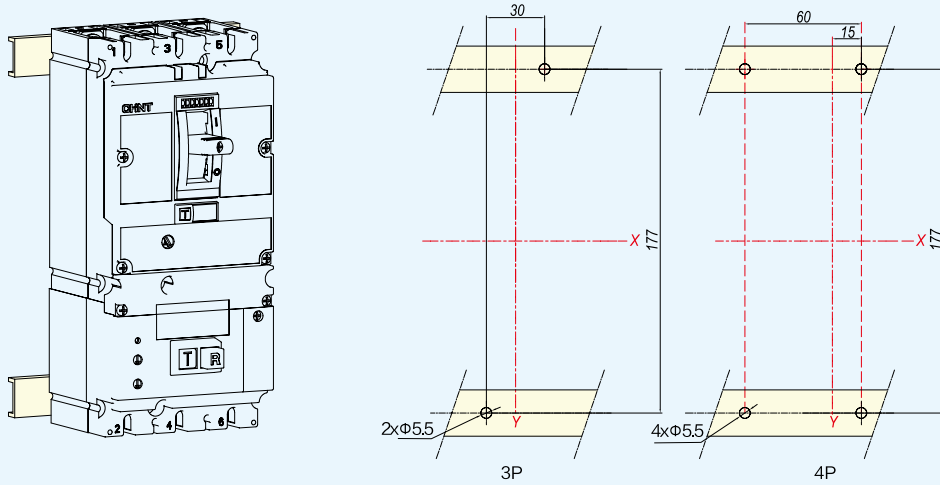
NM8NL-125 导轨安装
