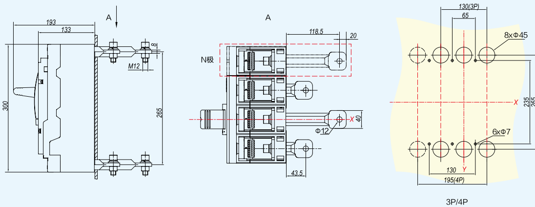
NM8N-800 板后连接
