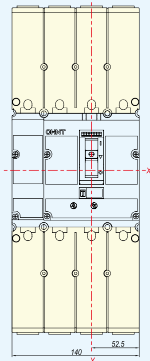
4P长端子罩
