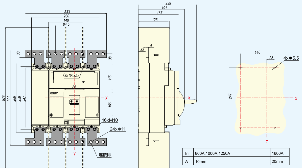
NM8N-1600 板前连接 (手动版 4P)
