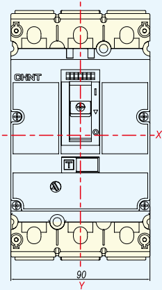
3P短端子罩
