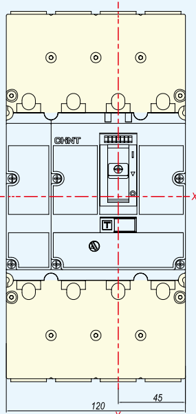
4P长端子罩
