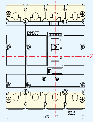
4P短端子罩
