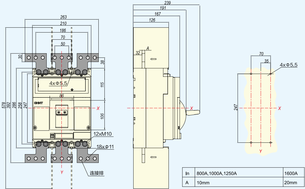
NM8N-1600 板前连接 (手动版 3P)
