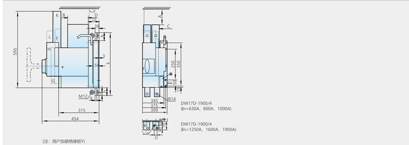
图 16-2 DW17D-1900/4(I n =630~1900) 四极固定式垂直接线
