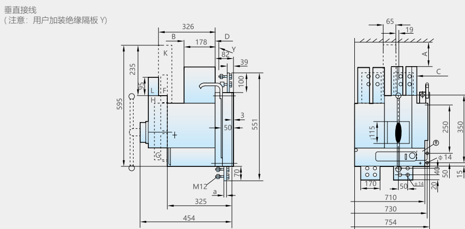
图 16-4 DW17D-2900/4(In=2000A~2500A) 四极固定垂直接线
