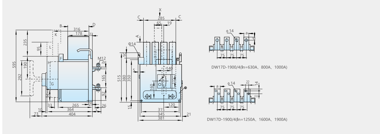
图 16-1 DW17D-1900/4(I n =630~1900) 四极固定式水平接线
