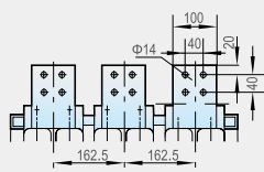
DW17D-2900(In = 2000A、2500A))
