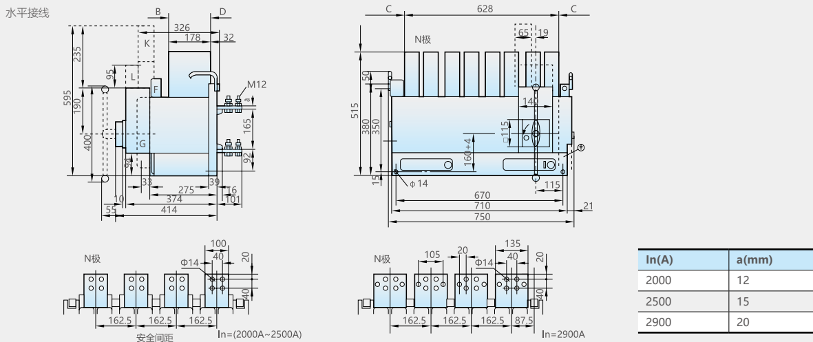
图 16-3 DW17D-2900/4(In=2000A~2900A) 四极固定水平接线
