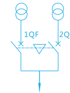
电路图
