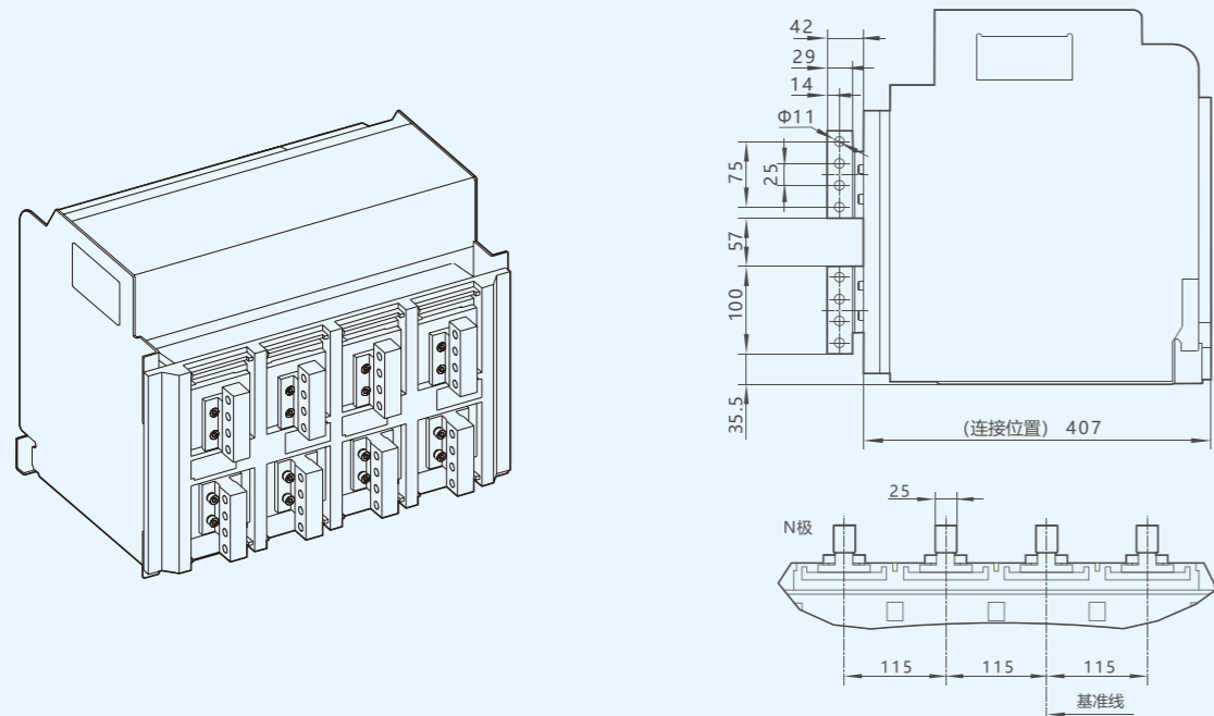
垂直连接 (In=3200A ~ 4000A) 侧视图
