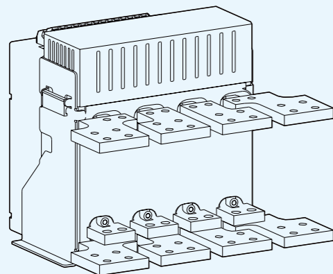
四极产品水平扩展母线（可选） 侧视图
