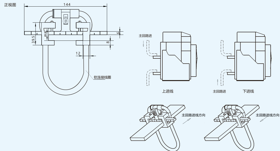
正视图
