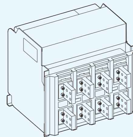
垂直连接 侧视图
