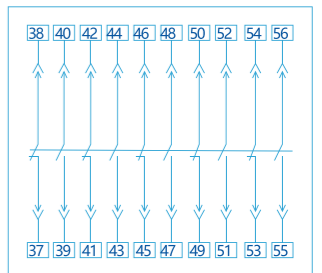
N4 四常开四常闭触头 (可选) N5 五常开五常闭触头 (可选)
