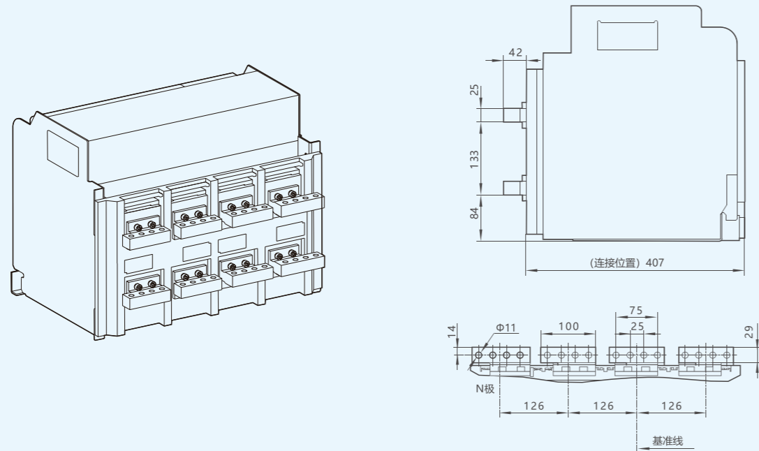
水平连接 (In=3200A ~ 4000A) 侧视图
