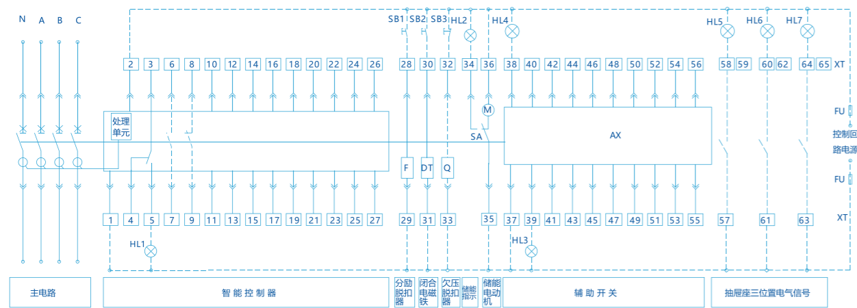
N3 三常开三常闭触头 (可选) N5 五常开五常闭触头 (可选)
