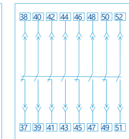
N4 四常开四常闭触头 (可选) N5 五常开五常闭触头 (可选)
