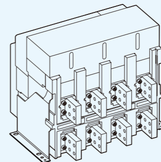
垂直连接 侧视图
