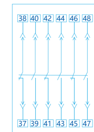
N3 三常开三常闭触头 (可选)
