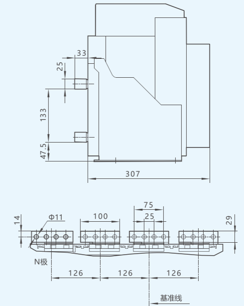
母排安装尺寸
