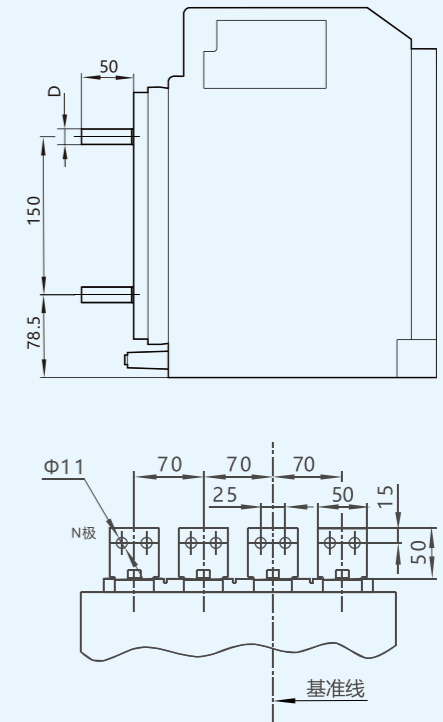
垂直连接 母排安装尺寸
