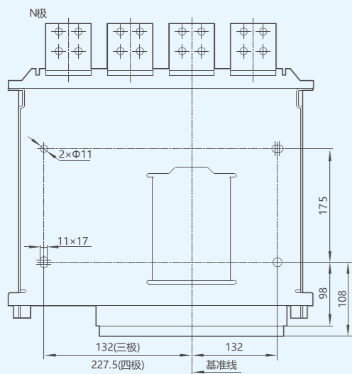
底座开孔尺寸
