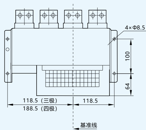
开孔尺寸 底座开孔尺寸
