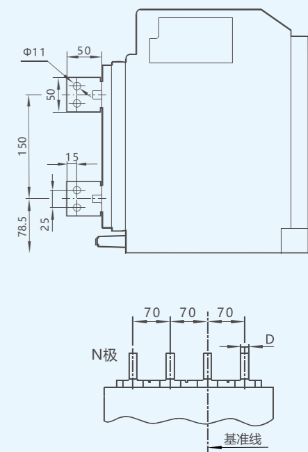
垂直连接 母排安装尺寸
