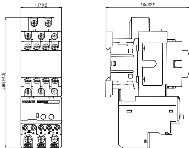
Ex9RE40+Ex9C09 - 18 Unit: in [mm]
