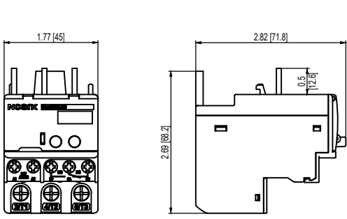
Ex9RE40 Unit: in [mm]
